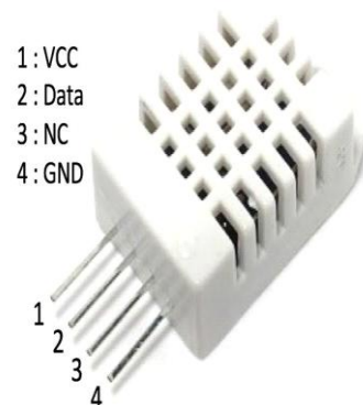
Fig. 2. DHT22
