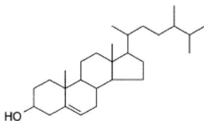
Sitosterol
