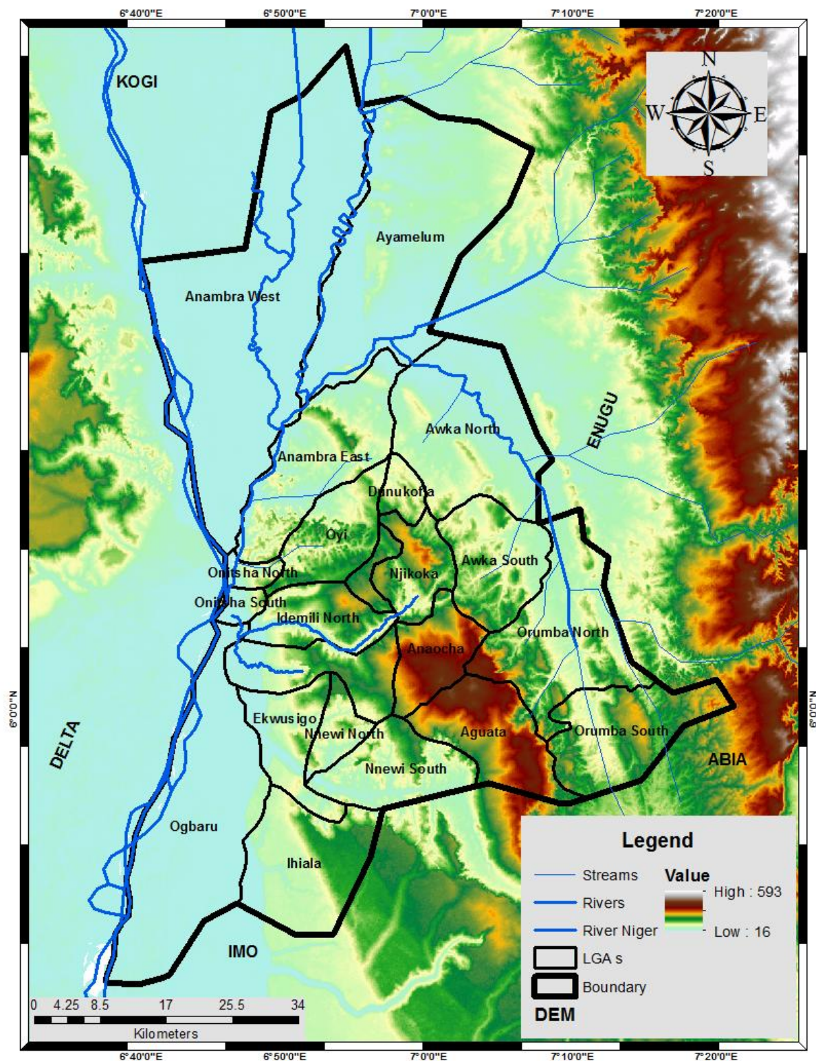
Fig 3a: Dem of Anambra State
