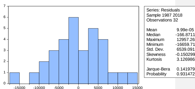
Fig. 5. Jarque-Bera test
