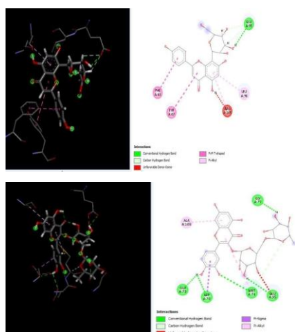
Vitexin -9.3
