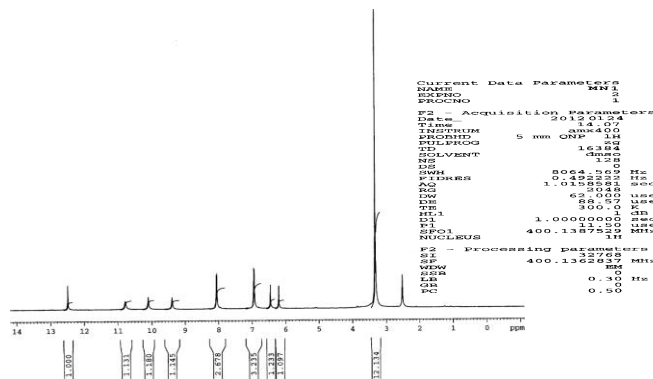
I-b ( ^1\text{H} NMR spectra)
