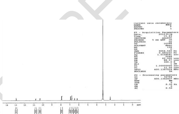
III-b ( 1 H NMR spectra)
