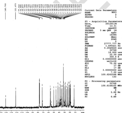
II-b (HNMR spectra)
