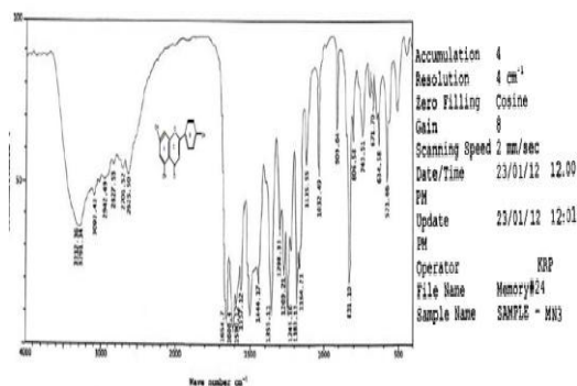
III-a (IR spectra)
