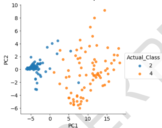
Fig. 4.2 Scatter plot of actual values (class) using PCA
