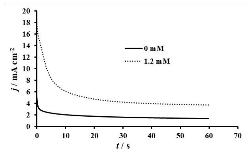
Figure 10. Courbes chronoampérométriques en milieu \text{H}_2\text{SO}_4 (0.1 M) pH = 9, en absence et en présence de 1.2 mM d'OMP
