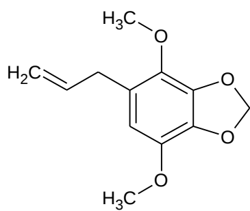
Apiol
