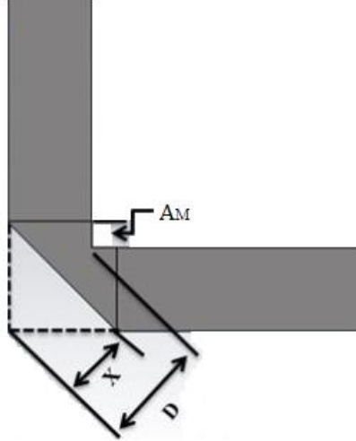
Fig.8. Microstrip mitred bend
